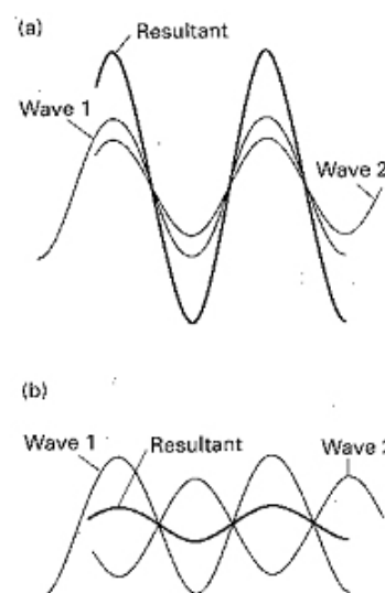
Figuur 17: Superpositie van golf functies
