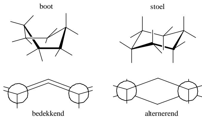
Figuur 51: Conformaties van cyclohexaan
