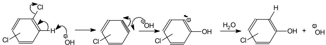
Figuur 65: Een alternatief mechanisme met benzyn als intermediair
