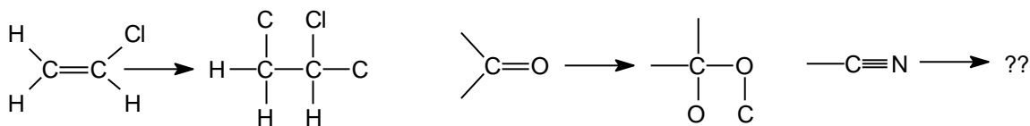
Figuur 54: Prioriteitenregel en dubbele bindingen
