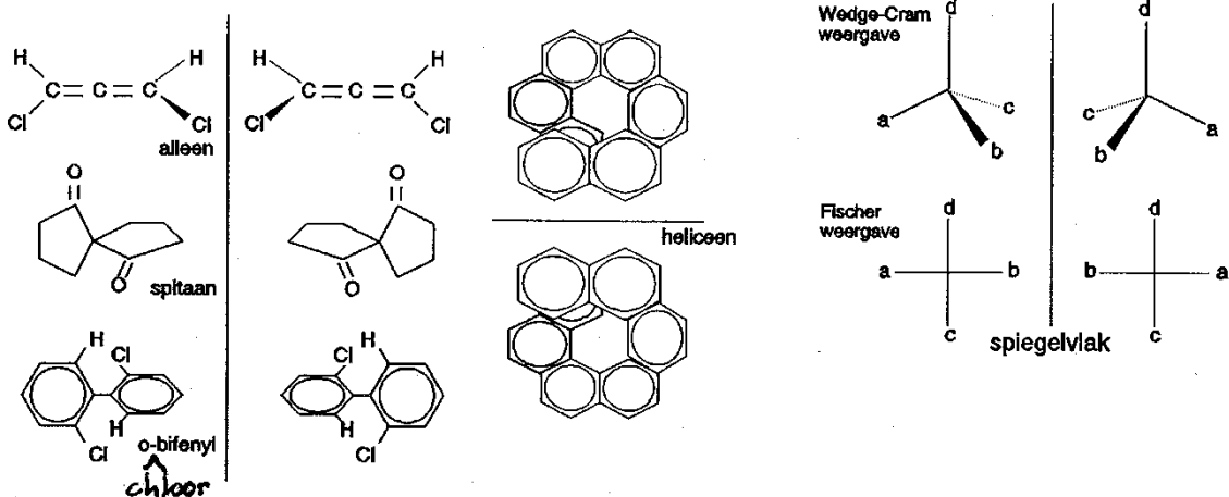
Figuur 60: Chirale moleculen
