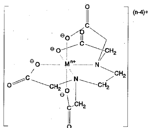
Figuur 38: Zestendig complex met EDTA
