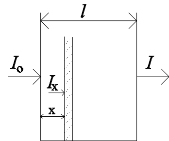
Figuur 70: Lambert-Beer
