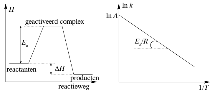
Figuur 48: Bepaling reactieconstante
