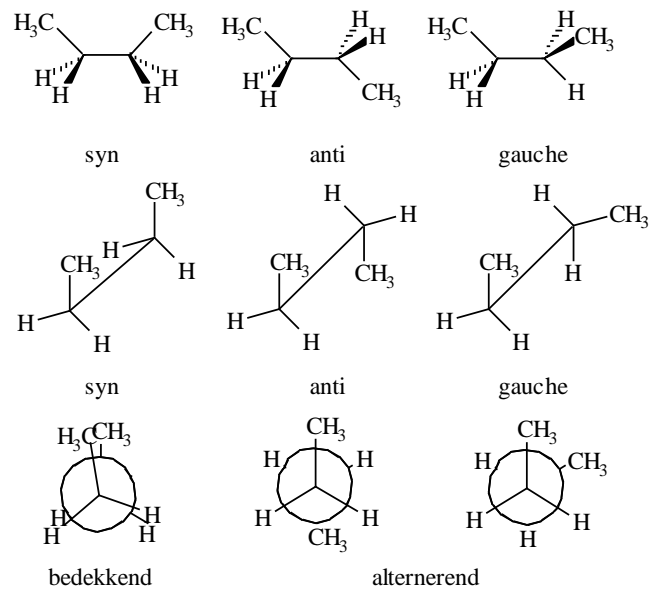
Figuur 50: Benamingen conformaties
