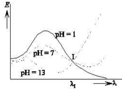
Figuur 71 Absorptiespectra van HIn
